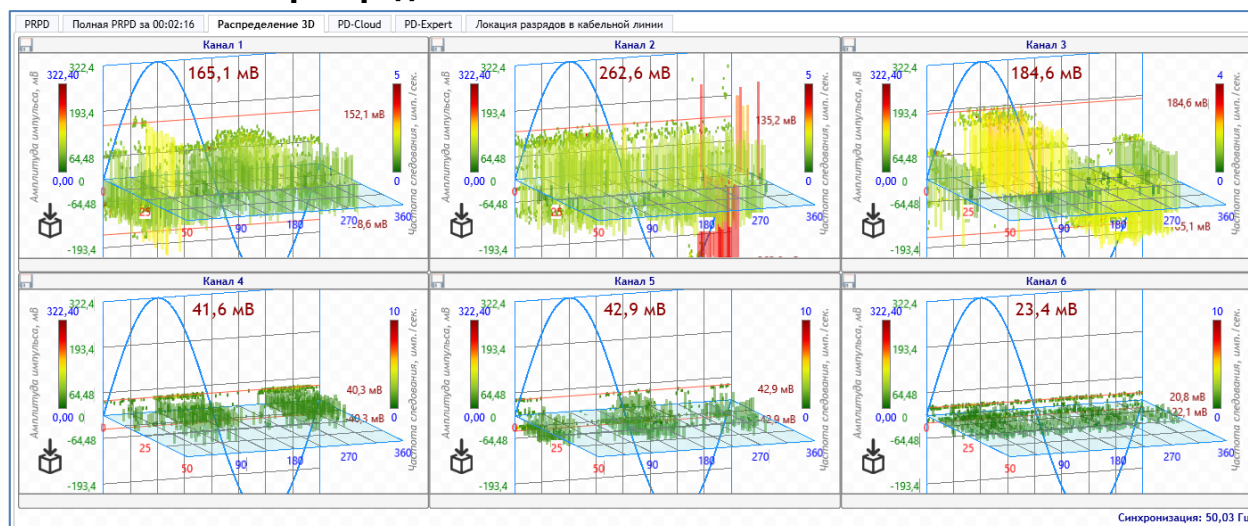
Рисунок 3.8 3D-распределение
