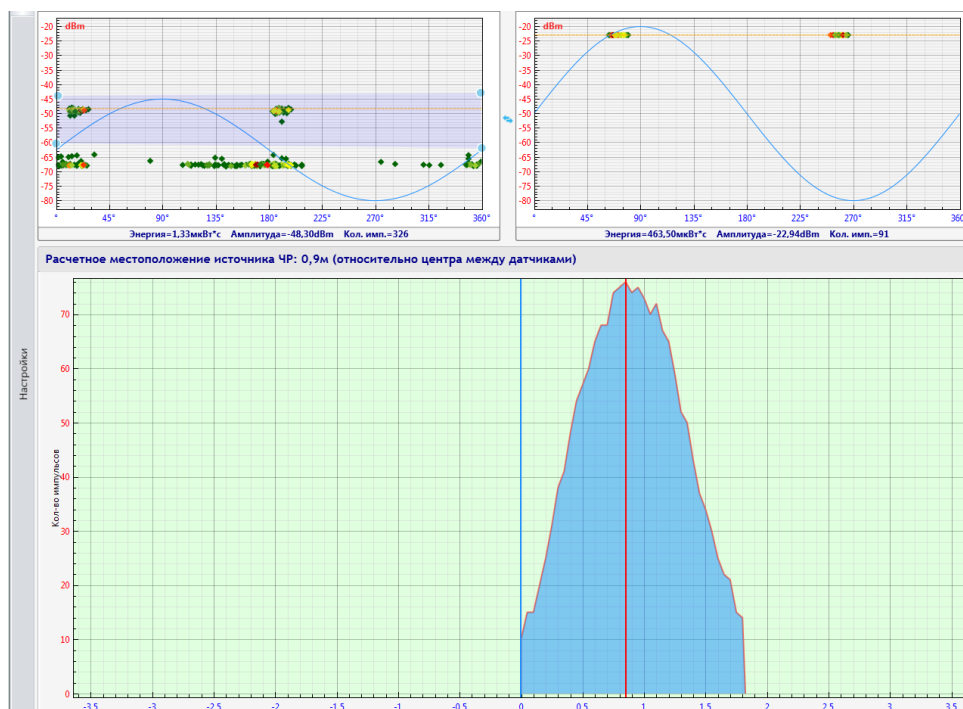
Рисунок 3.15 Окно локации разрядной активности.
