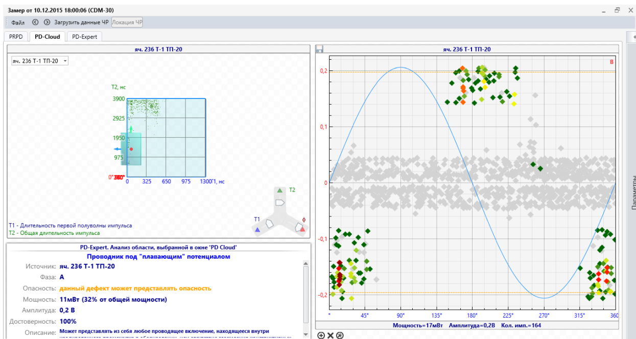
Рисунок 3.9 PD-Cloud
