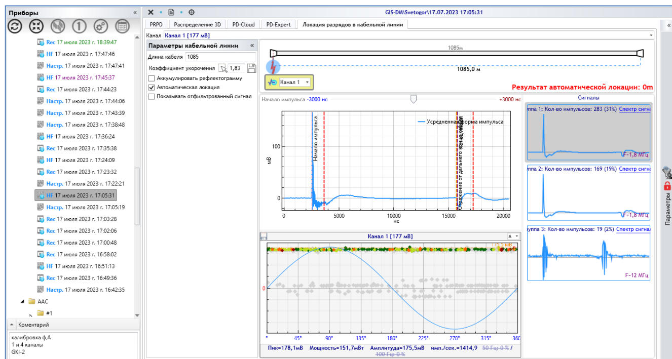
Рисунок 3.11 Локация разрядов в кабельной линии
