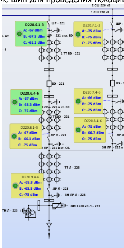
Рисунок 3.13 Схема КРУЭ с выбранными для локации датчиками.
