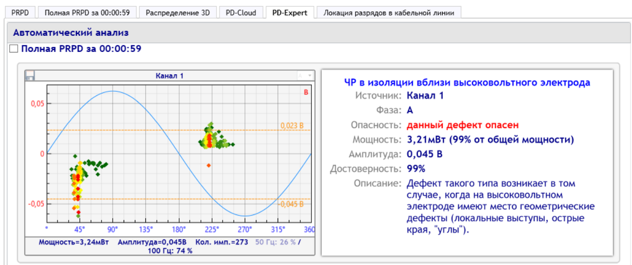
Рисунок 3.10 PD-Expert
