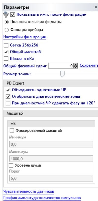
Рисунок 3.17. Панель «Параметры»
