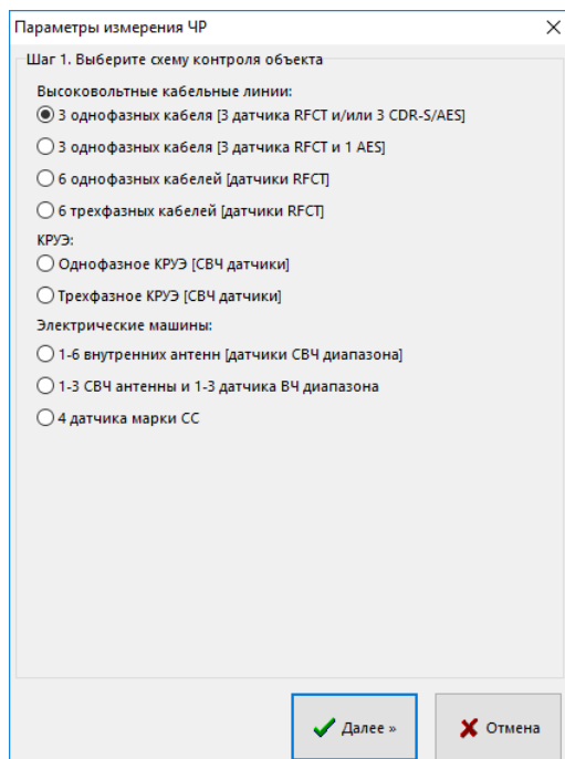
Рисунок 3.4 Помощник настройки
