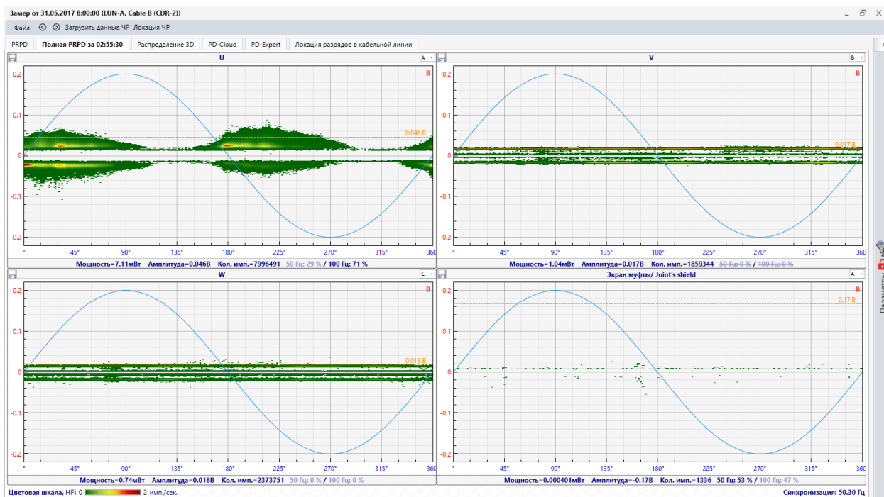
Рисунок 3.7 Полная PRPD
