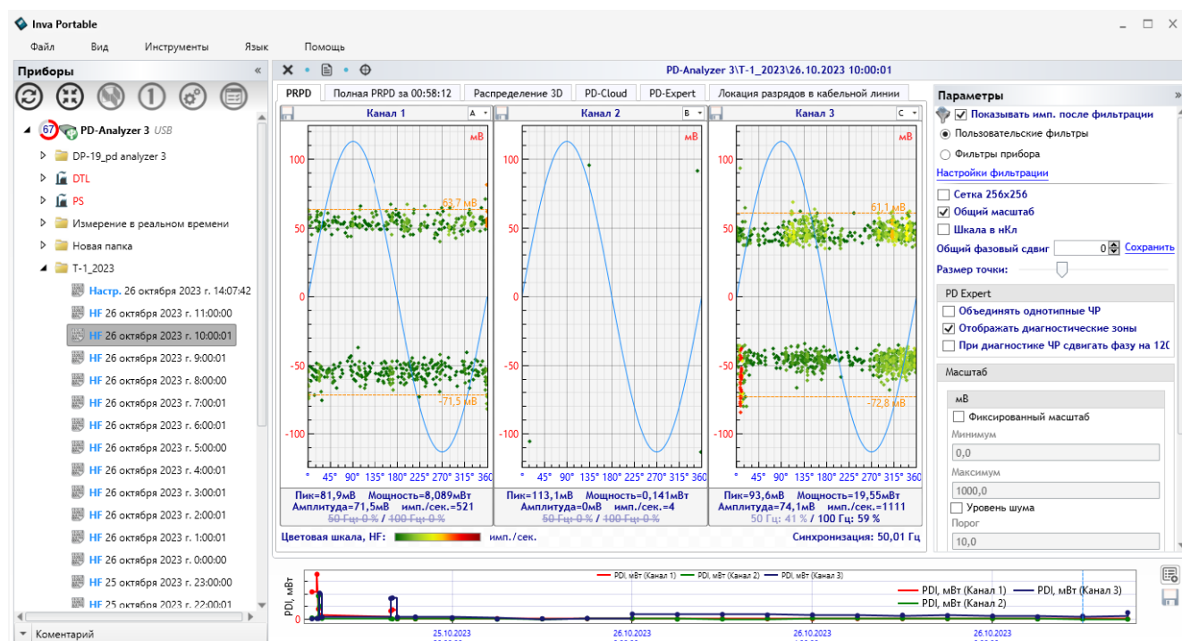
Рисунок 40. Просмотр тренда и амплитудно-фазового распределения ЧР PRPD
