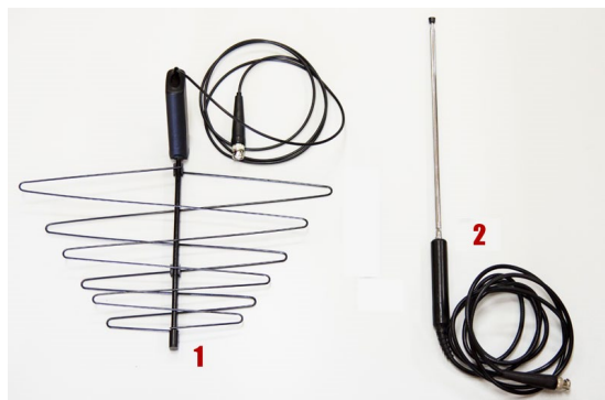
Рисунок 10. СВЧ антенны
