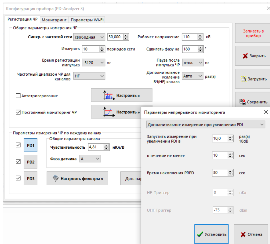
Рисунок 33. Настройки параметров непрерывного мониторинга
