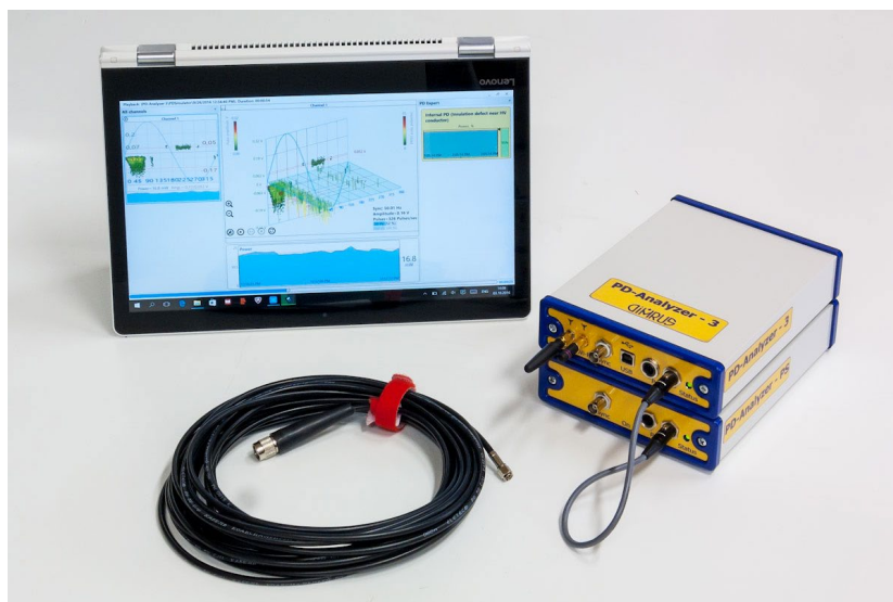
Рисунок 1. Внешний вид прибора «PD-Analyzer/3P»
