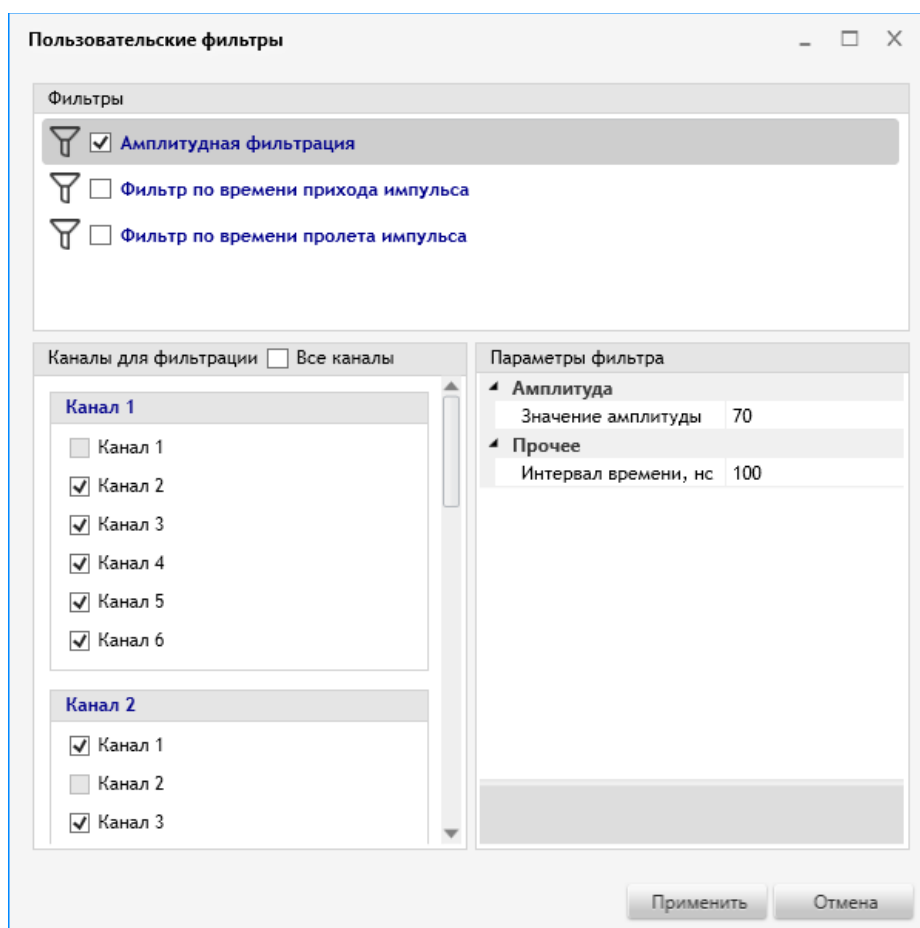
Рисунок 51. Окно настройки фильтрации импульсов
