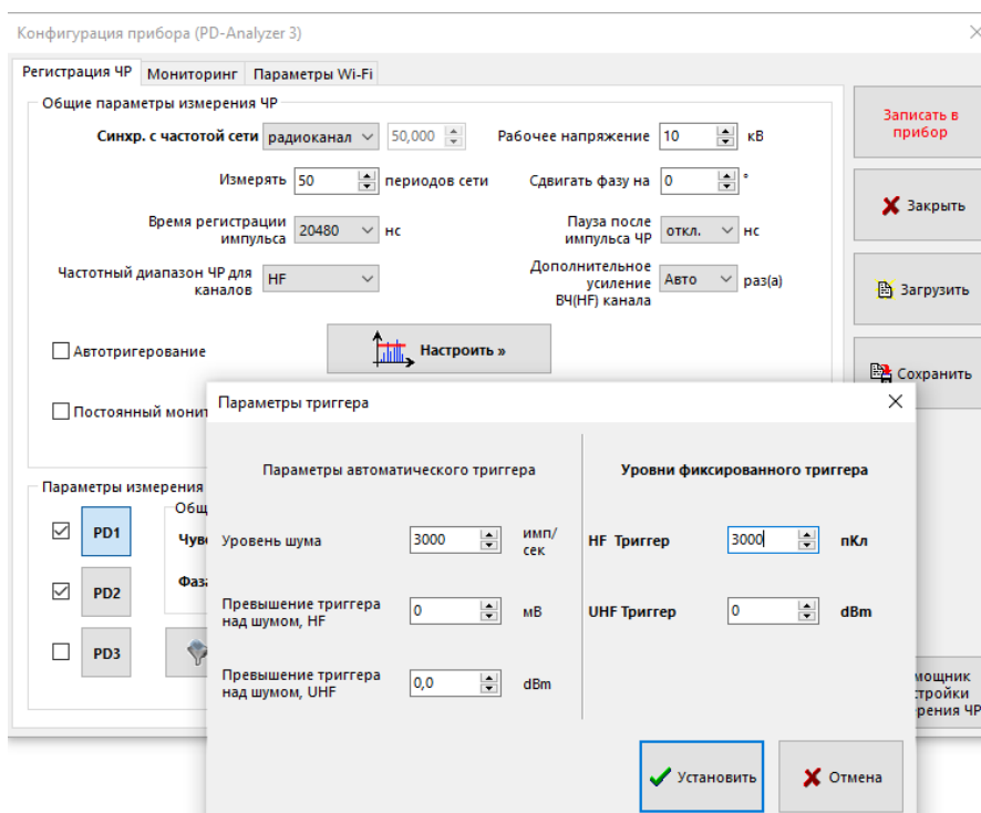
Рисунок 32. Настройки параметров фиксированного триггера
