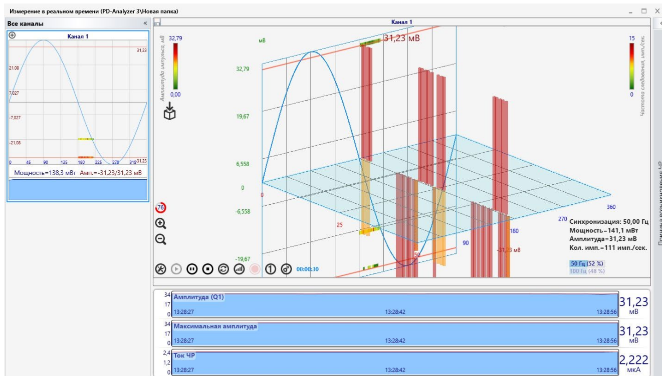
Рисунок 38. Измерение в режиме реального времени
