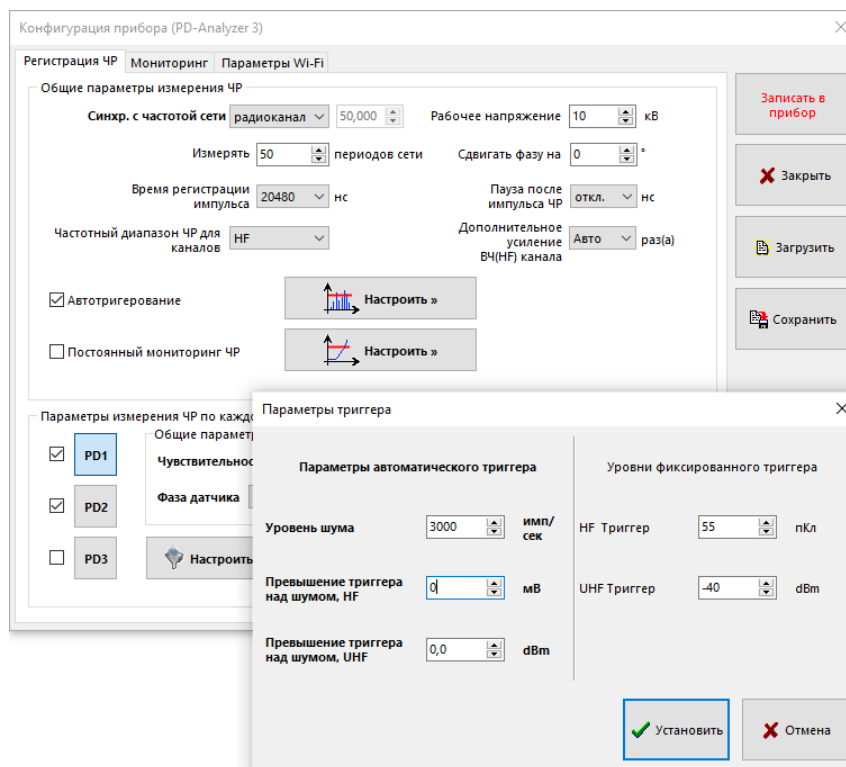
Рисунок 31. Настройки параметров автоматического триггера
