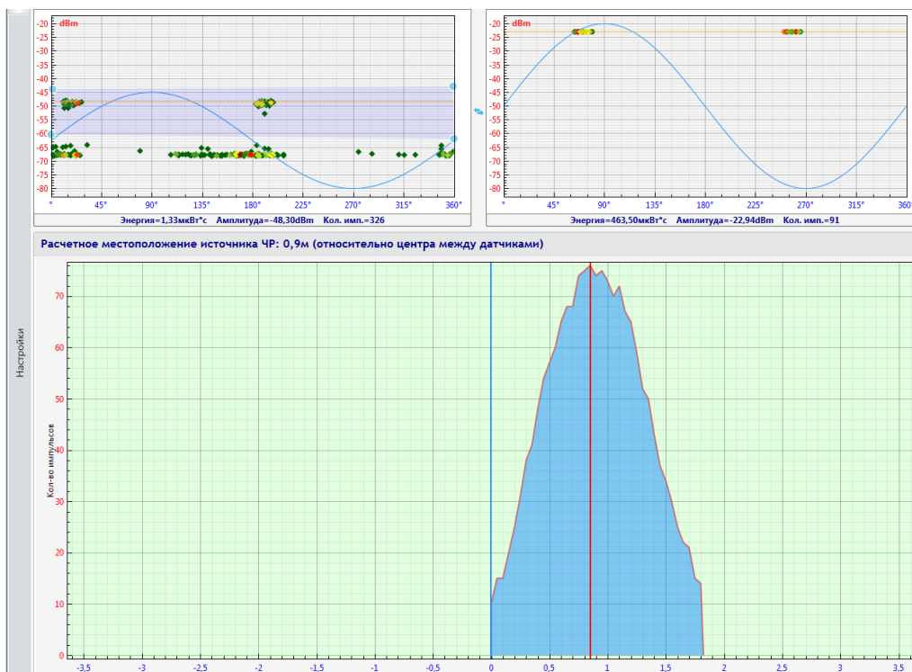
Рисунок 48. Окно локации разрядной активности
