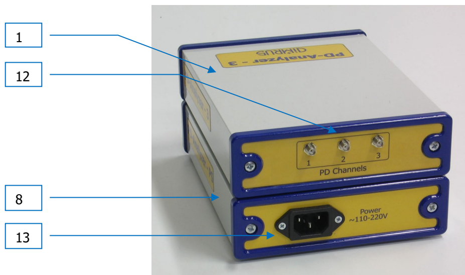
Рисунок 3. Тыльная панель прибора
