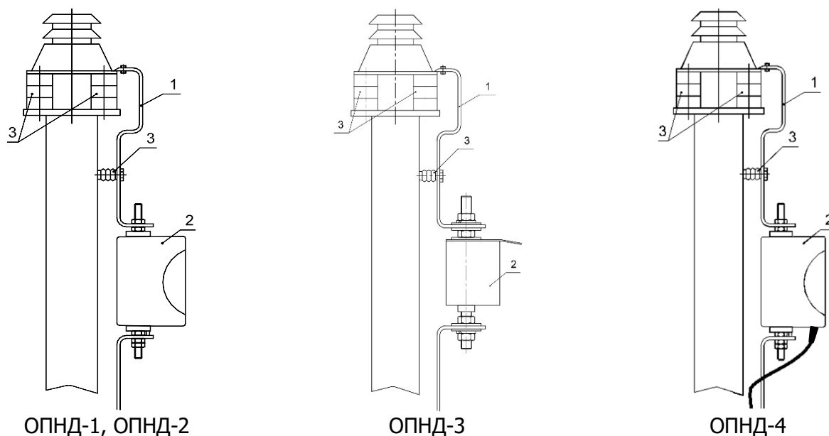
Рисунок 2 – Схема размещения и подключения датчиков:
