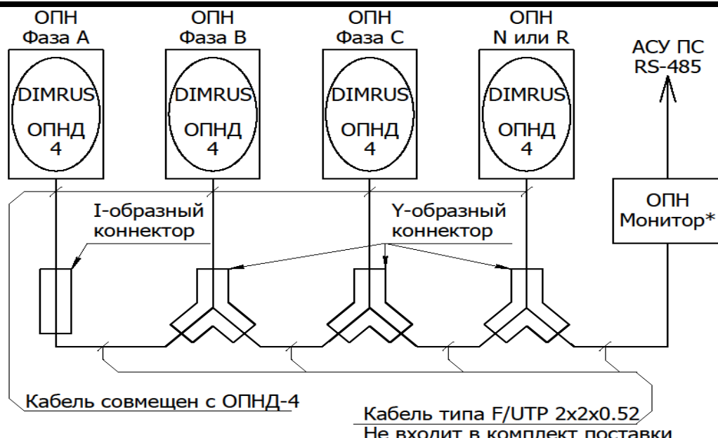
Рисунок Г.2 – Вариант подключения датчиков ОПНД-4 с помощью прибора ОПН-Монитор.
