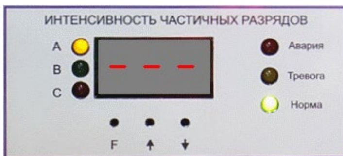
Рисунок 4. Вид индикаторов во время измерения уровня ЧР
