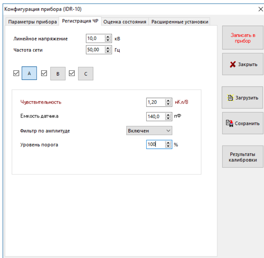
Рисунок 27. Регистрация ЧР
