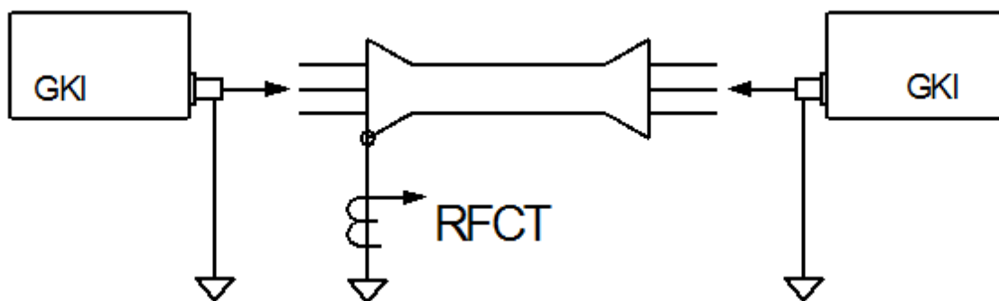
Рисунок 31. Калибровка в кабельной линии
