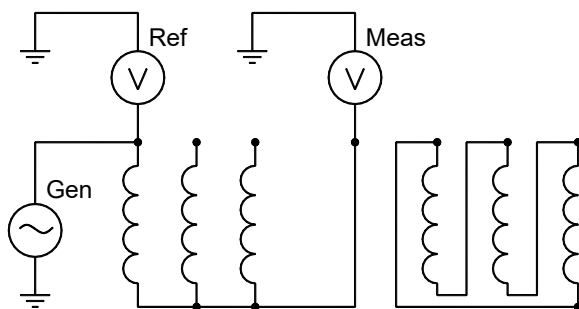
Рисунок 5.1. Схема A-N [Open]
