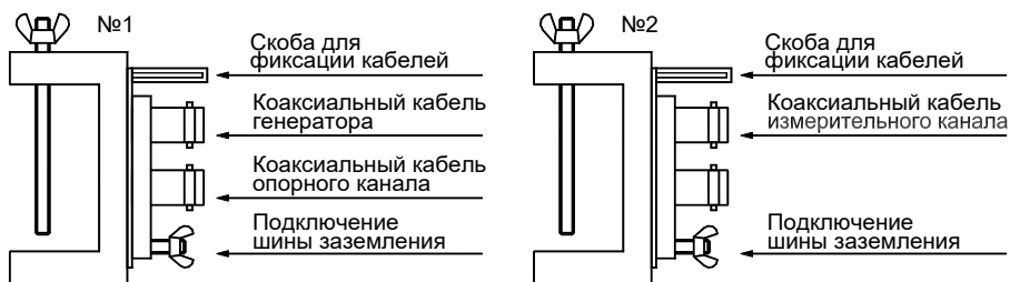
Рисунок 3.2. Струбцины для подключения
