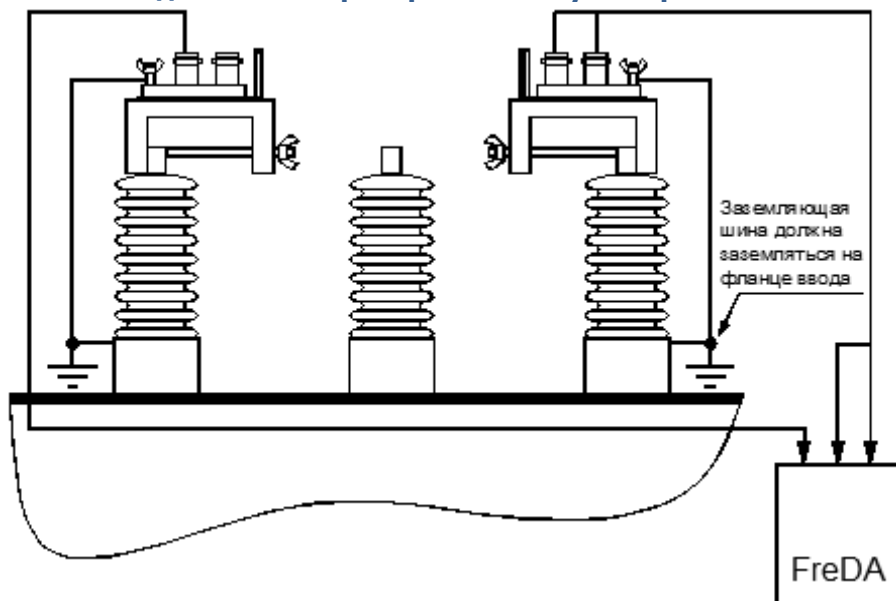
Рисунок 3.1. Подключение прибора к объекту
