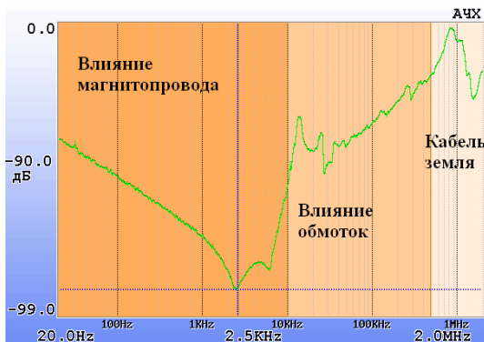
Рисунок 2.2. Проявление дефектов в диапазонах частот
