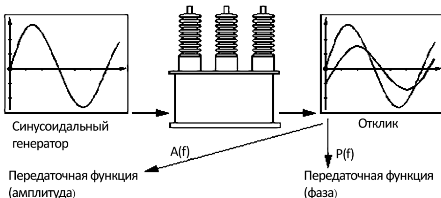
Рисунок 2.1. Метод частотного анализа
