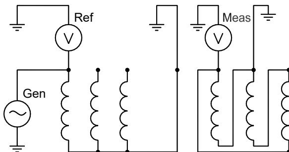
Рисунок 5.4. A-a1 [IIW, GND N,n1]
